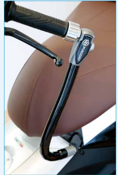
605537M013 Diebstahlsicherung dient zur einfachen, schnellen und zusätzlichen Sperre des Lenkers. Sie wird direkt unter der Sitzbank und einer zusätzlichen Vorrichtung am Lenker montiert. Bei Nichtnutzung verbleibt sie direkt am Fahrzeug, wobei hier z.B. ein Helm befestigt werden kann.
